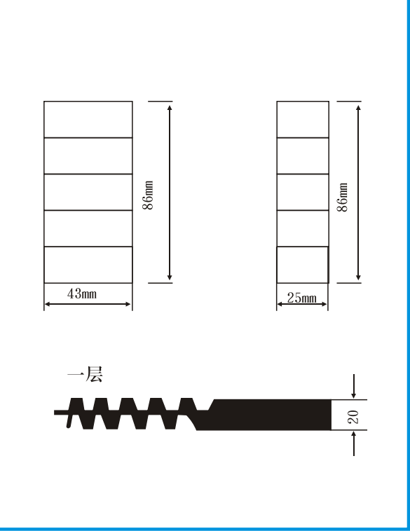
SD型隔振垫0.5基本块尺寸
